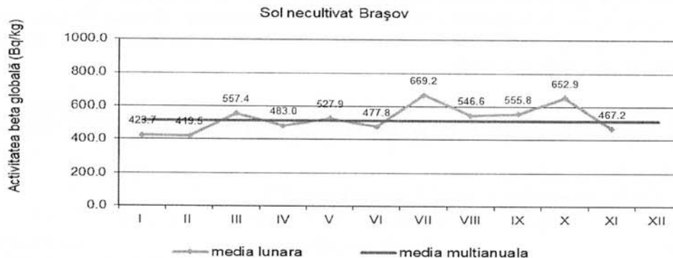
Fig. 1.2.8. Activitatea beta globală la 5 zile pentru sol necultivat
