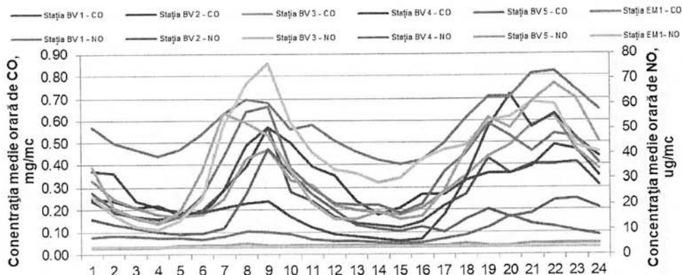
Figura 1.1.2.2.4. Ciclul zilnic al NO și CO
