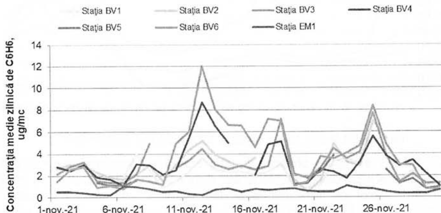
Figura 1.1.2.6.1: Evoluția mediilor zilnice de benzen în luna noiembrie
