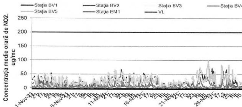
Figura 1.1.2.2.1. Evoluția mediilor orare de NO 2 în luna noiembrie
