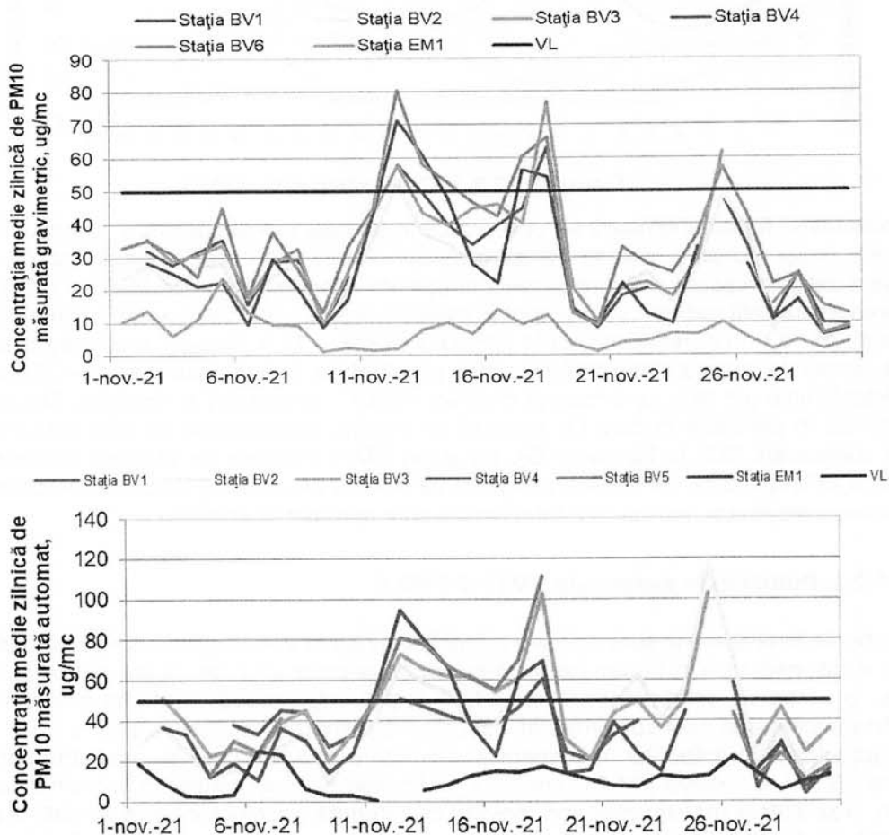
Figura 1.1.2.4.1. Evoluția mediilor zilnice de PM 10 în luna noiembrie
