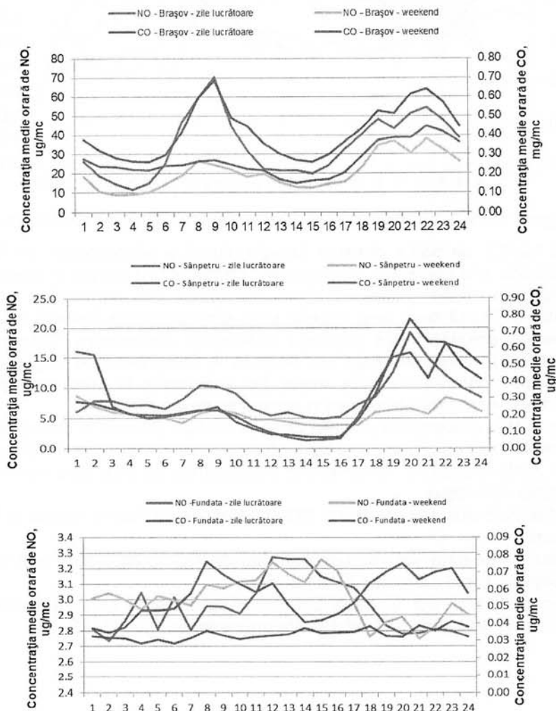
Figura 1.1.2.2.5. Ciclul zilnic al NO și CO în timpul săptămânii
