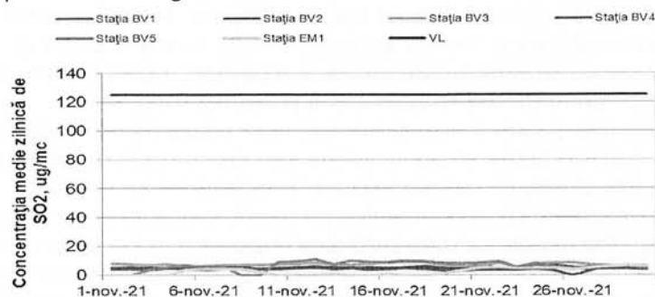
Figura 1.1.2.1.1. Evoluția mediilor zilnice de \text{SO}_2 în luna noiembrie
