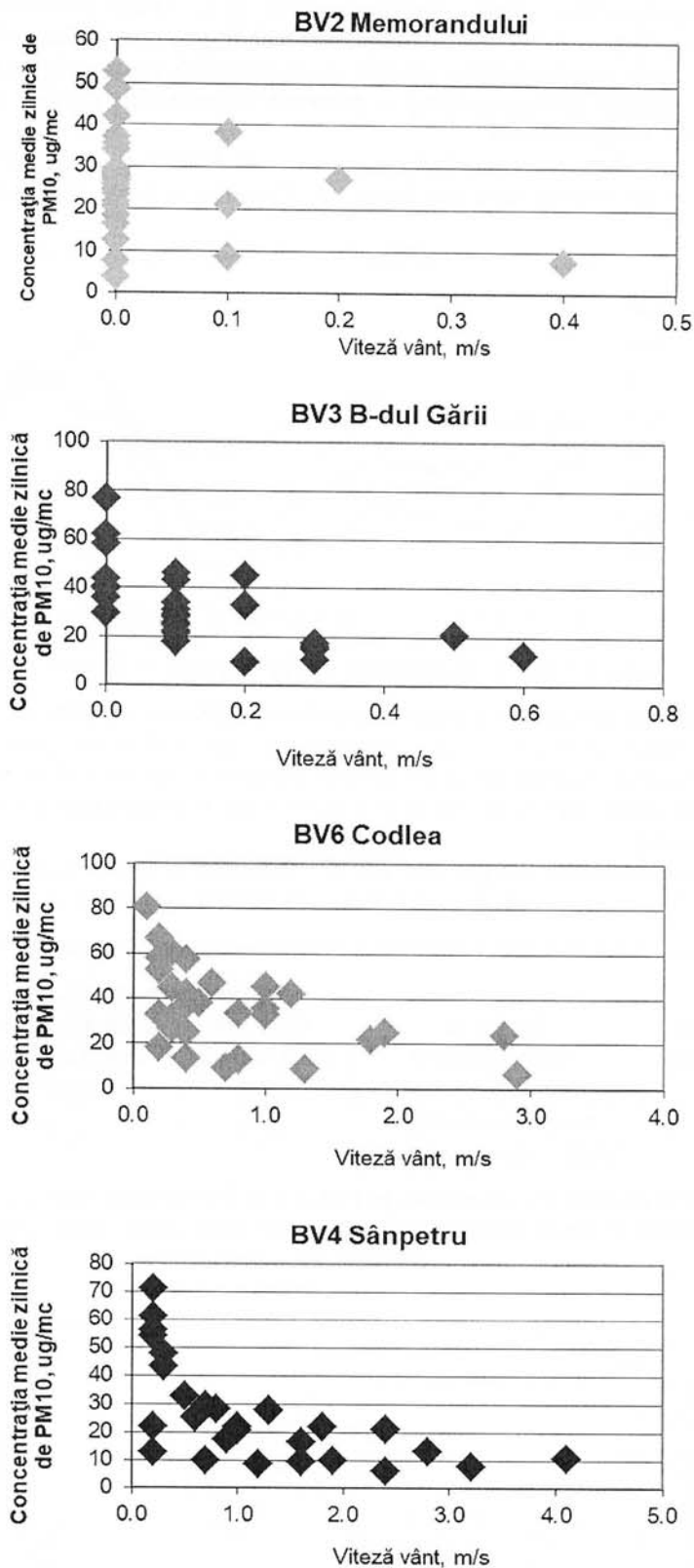
Figura 1.1.2.4.2. Evoluția mediilor zilnice de PM 10 în funcție de viteza vântului
