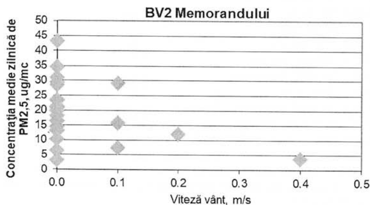
Figura 1.1.2.4.5. Evoluția mediilor zilnice de \text{PM}_{2,5} în funcție de viteza vântului
