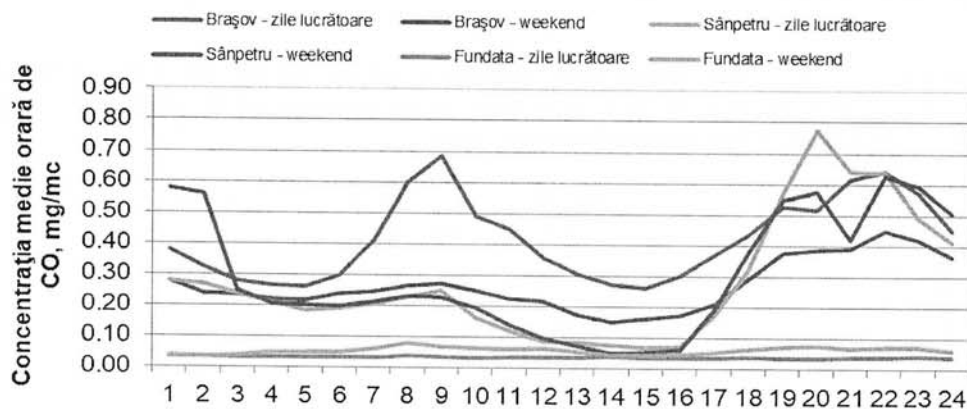
Figura 1.1.2.5.3. Ciclul zilnic al CO în timpul săptămânii
