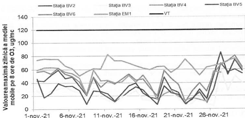
Figura 1.1.2.3.1. Evoluția maximelor zilnice ale mediilor mobile pe 8 ore de O 3 în luna noiembrie
