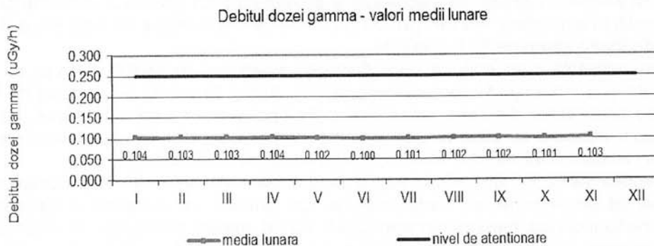
Fig. 1.2.3. Debitul dozei gamma în aer
