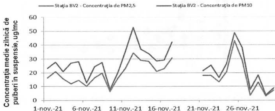
Figura 1.1.2.4.4 Evoluția mediilor zilnice de PM 2,5 și PM10 în luna noiembrie
