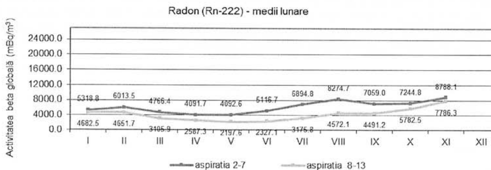
Fig. 1.2.2. Activitatea calculată a Radonului
